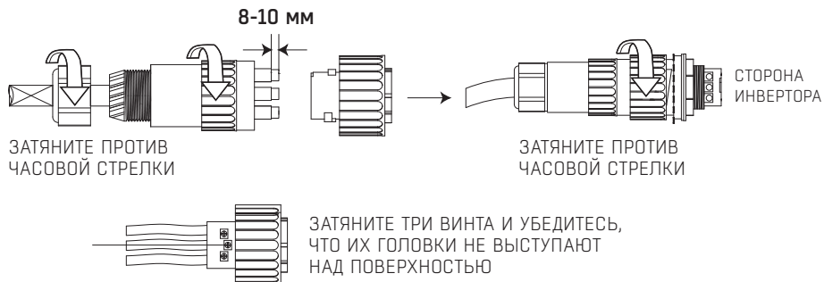
Рисунок 3.4.3.1. Инструкция по монтажу кабелей
